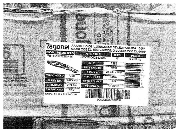
Detalhe das especificações técnicas das luminárias LED em conformidade com o exigido no Edital
