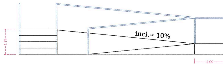
vista lateral RAMPA
