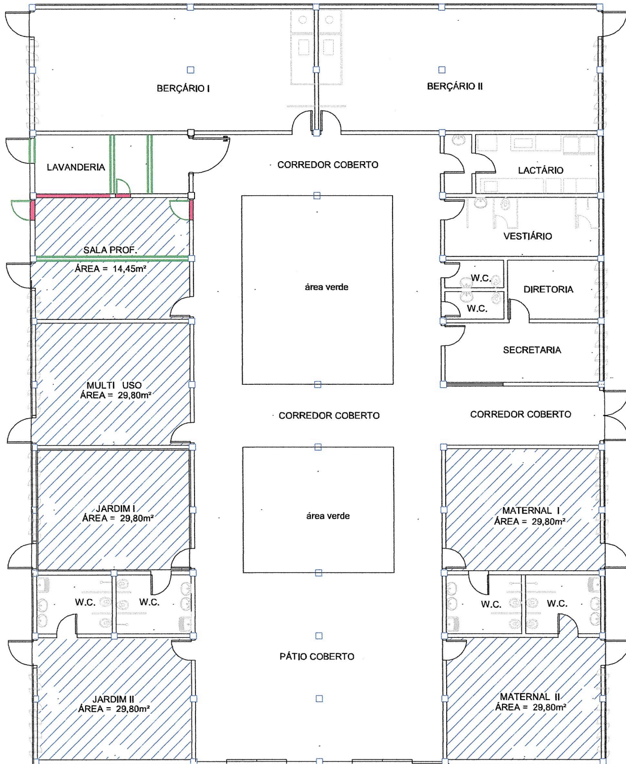
PLANTA BAIXA
