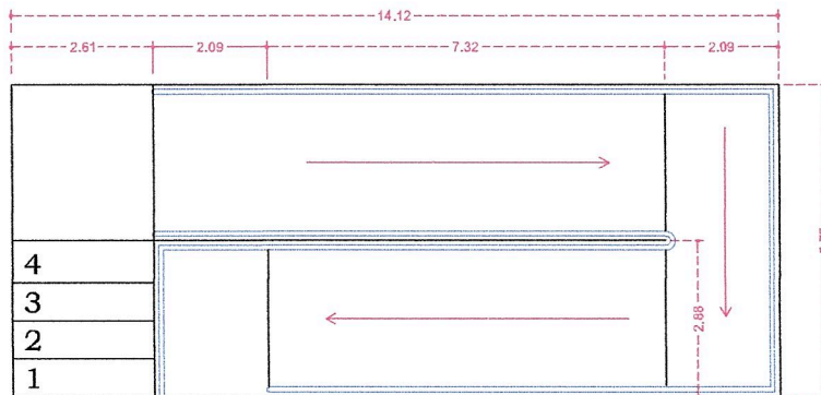
planta baixa - RAMPA
